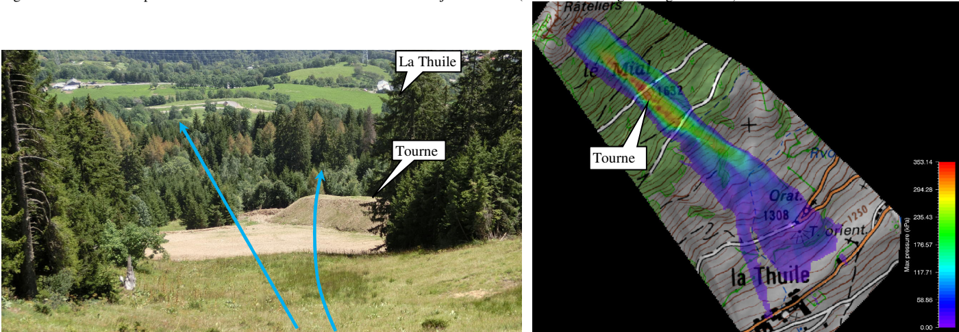
Fig.14 : trajectoires de l'avalanche du Mial au contact de la tourne.
